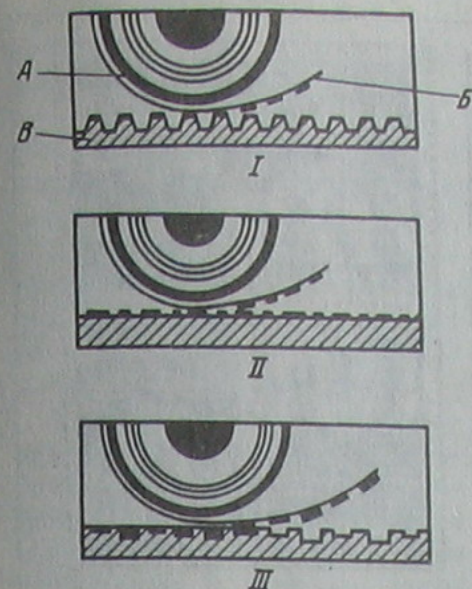
Рис. 1. Схемы основных способов печати: I — высокая; II — плоская; III — глубокая. А — цилиндр; Б — бумага; В — печатная форма.
